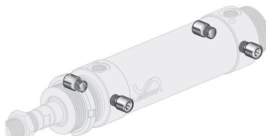
PIVOT FOR FLOATING HINGE MOUNTING PERNI PER MONTAGGIO A CERNIERA OSCILLANTE
